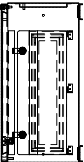
VUE DU BAS TRAPPE POUR ENTRÉE DE CÂBLES BOTTOM VIEW TRAP DOOR FOR CABLES
