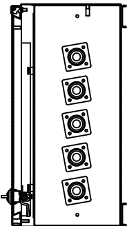
VUE DU BAS CONNECTEURS CAM LOK (SEULEMENT 5 MONTRÉS) BOTTOM VIEW CAM LOK CONNECTORS (ONLY 5 SHOWN)
