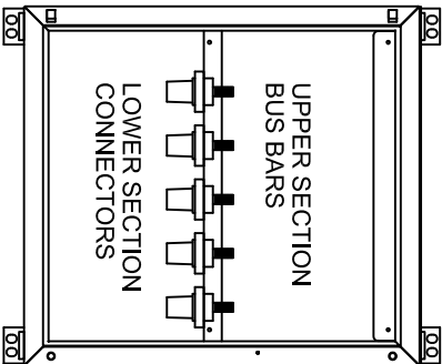
VUE AVANT CONNECTEURS CAM LOK (SEULEMENT 5 MONTRÉS) FRONT VIEW CAM LOK CONNECTORS (ONLY 5 SHOWN)
